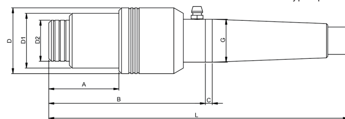
65型大子 65 type tips
