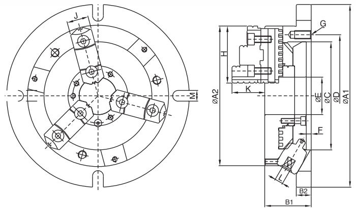
尺寸圖 / DIMENSIONS
