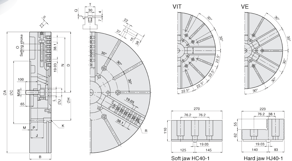
產品示意圖
